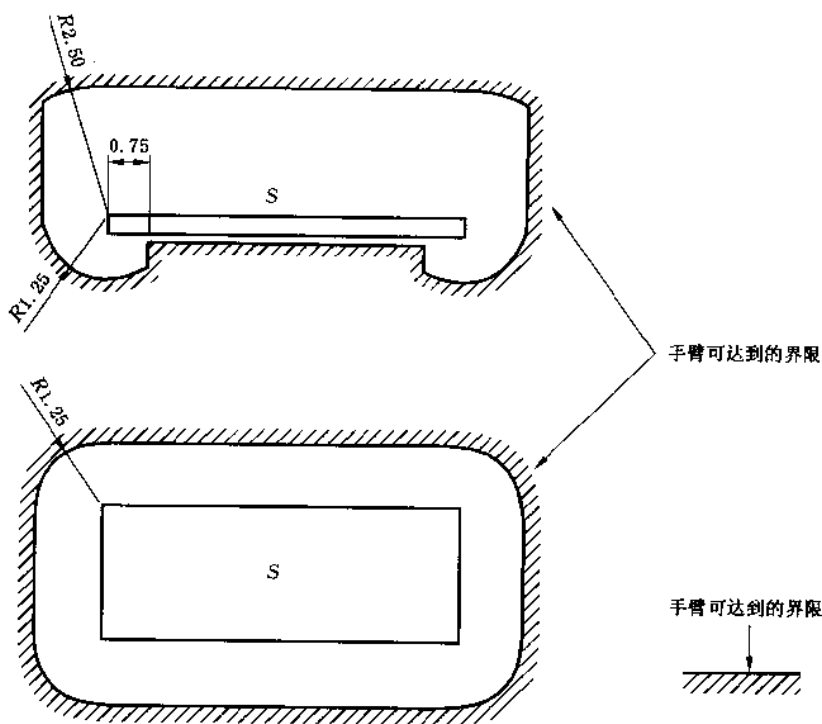
图 41C 伸臂范围
