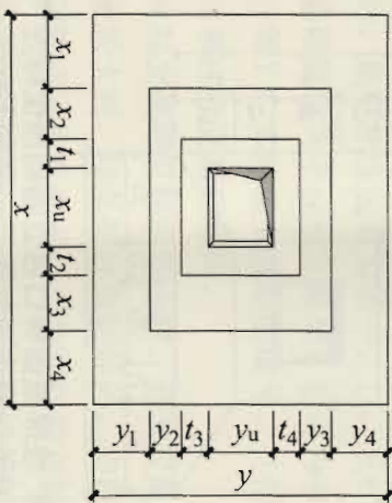
图 2.3.3-6 阶形截面杯口独立基础原位标注 (一)
