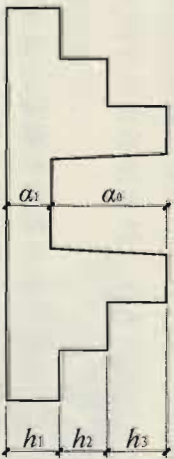
图 2.3.2-4 阶形截面杯口独立基础竖向尺寸 (一)
