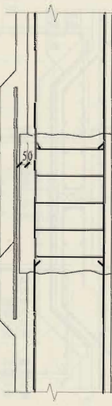
筏形基础 标准构造详图
