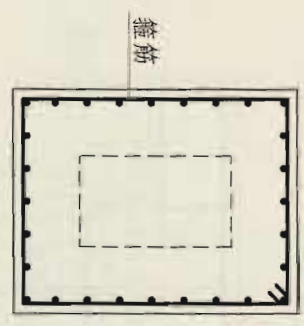
(矩形截面)
