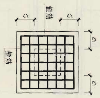
(正方形截面)
