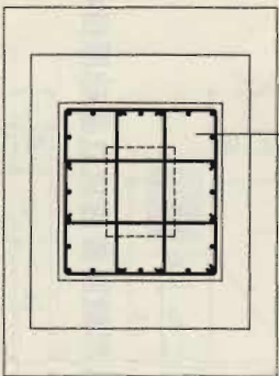
图 2.3.2-13 高杯口独立基础杯壁配筋示意
