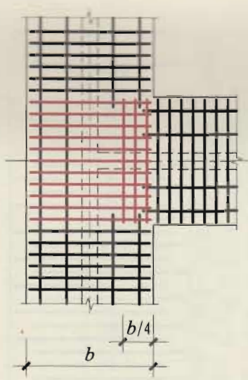
(丁字交接基础底板)
