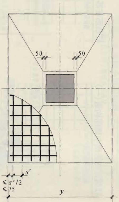
(b) 坡形
