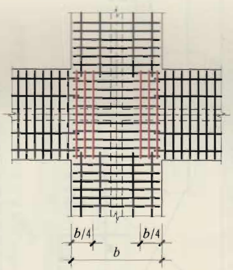
(十字交接基础底板)
