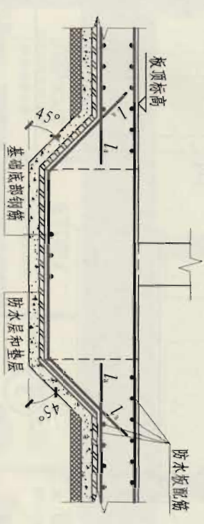
桩基承台 标准构造详图
