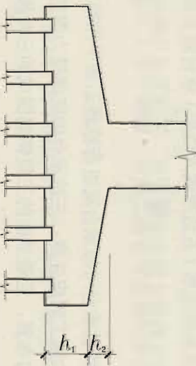
图 6.3.2-2 单阶截面独立承台竖向尺寸
