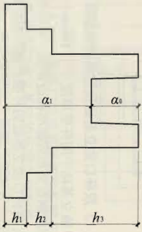
图 2.3.2-5 阶形截面杯口独立基础竖向尺寸 (二)
