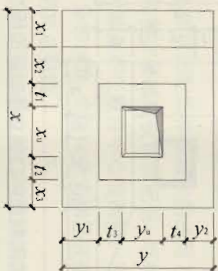
图 2.3.3-7 阶形截面杯口独立基础原位标注 (二)
