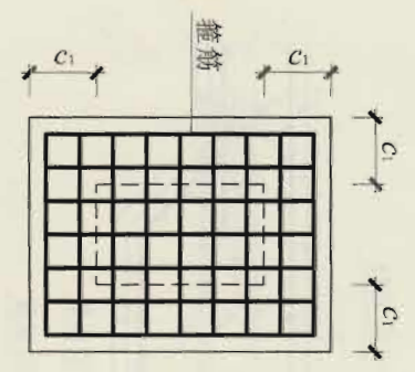
(矩形截面)
