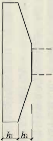
图 2.3.2-2 单阶普通独立基础竖向尺寸
