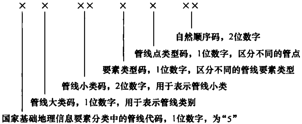
图 7.2.5 管线要素编码结构
