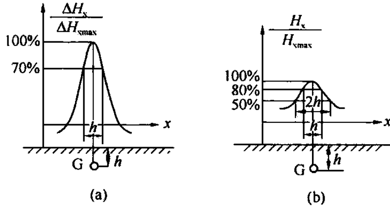
图2 电磁感应法管线定深示意
