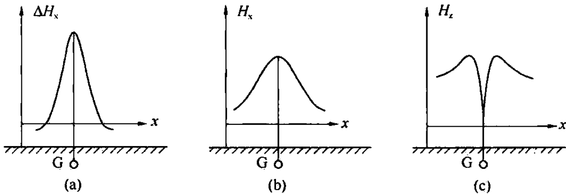
图 1 电磁感应法管线定位示意
