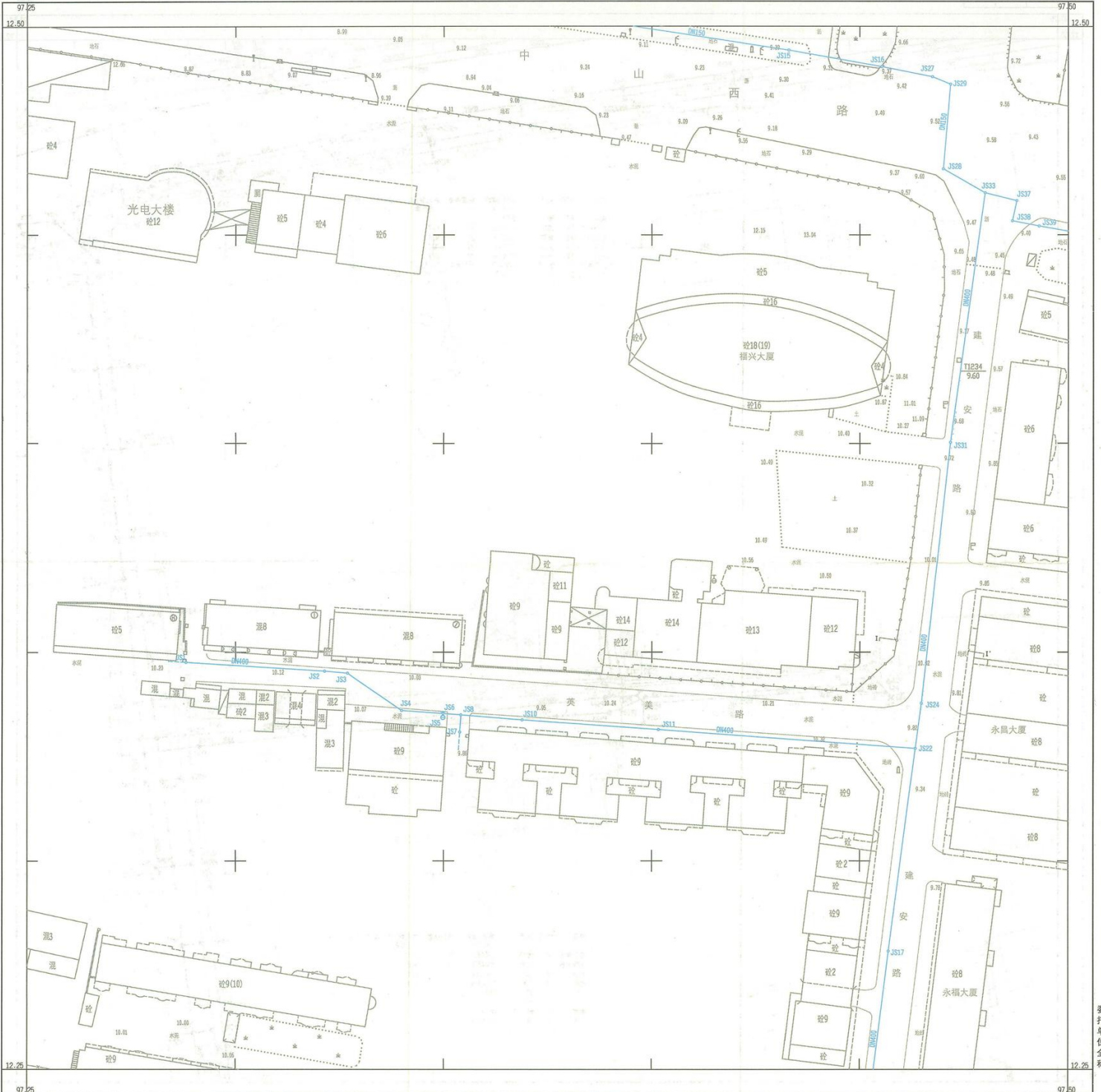
图 J-2 专业地下管线图样
