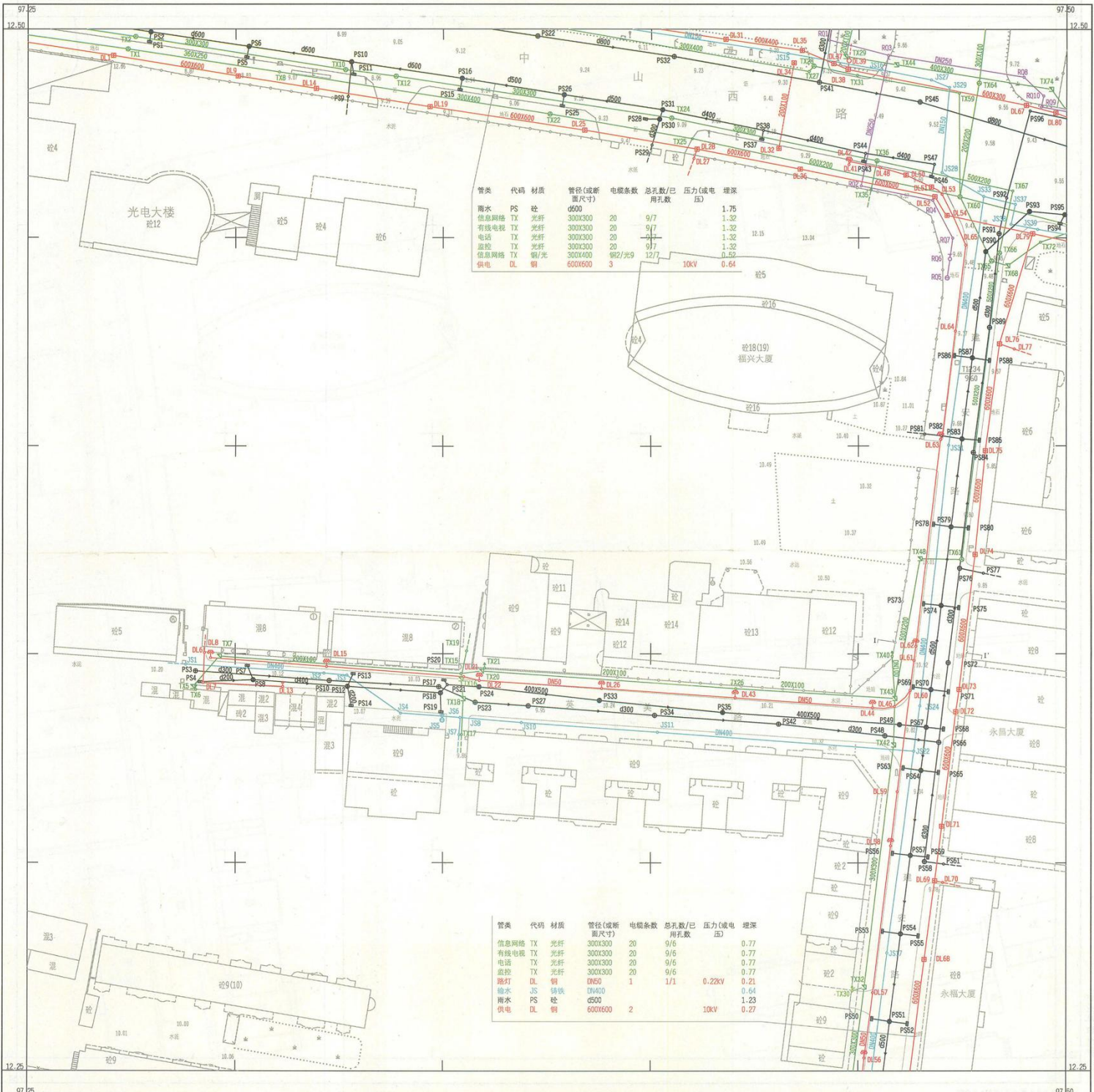
图 J-1 综合地下管线图样
